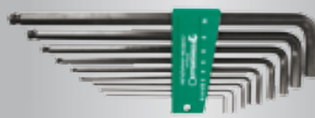
Zestaw kluczy trzpieniowych z końcówką kulistą (9-cz.) ● Nr 10767: 1,5; 2; 2,5; 3; 4; 5; 6; 8; 10 mm
